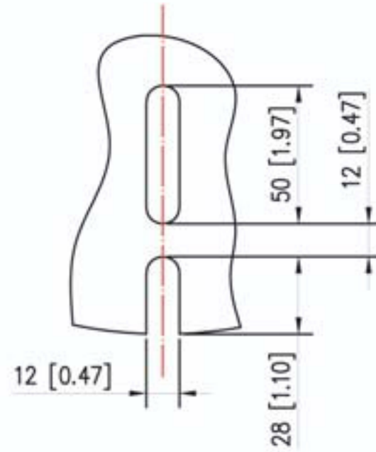
A-swivel
